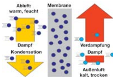
Funktionsschema Feuchterückgewinnung
