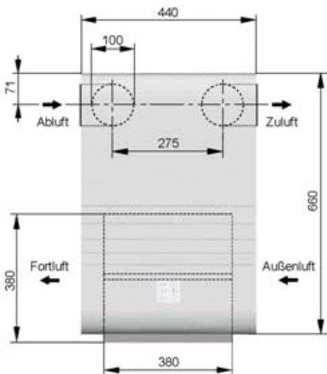
CA 70 mit Wandeinbaurohr WER R-CA 70
