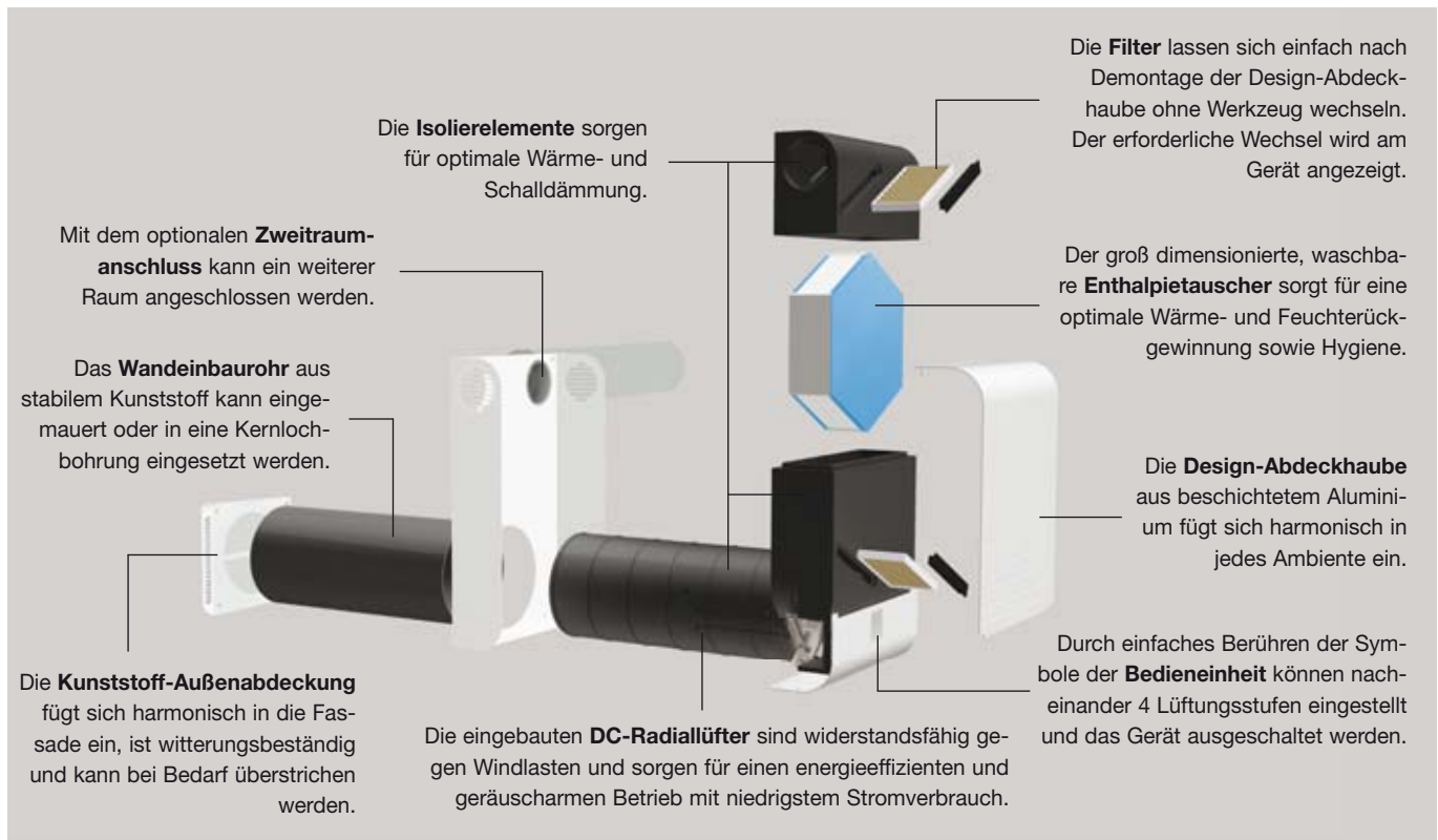
CA 70 mit Wandeinbaurohr WER R-CA 70
