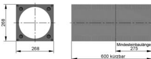
Wandeinbaurohr quadratisch WER Q-CA 70
