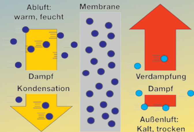
Schema: Wirkungsweise Enthalpietauscher
